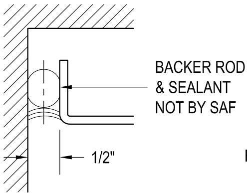
1 JAMB DETAIL
