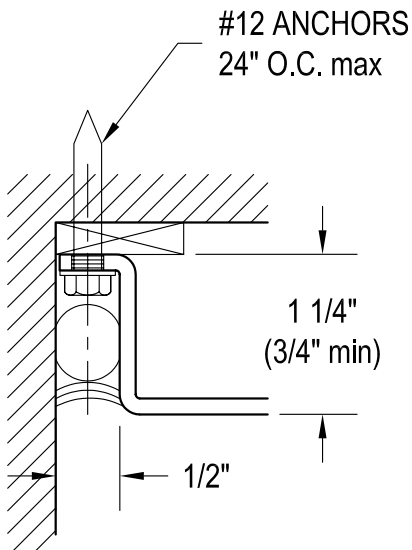
3 JAMB DETAIL
